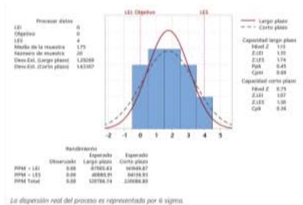
Fig. 15 Gráfica Six Sigma - CR-3 Nota. Muestra el informe de capacidad del proceso de errores de fabricación por día.
