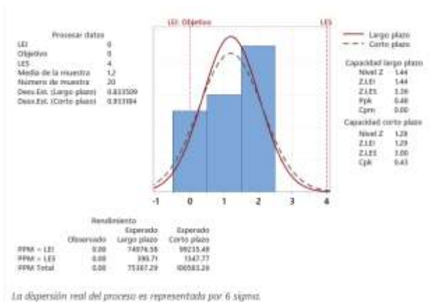
Fig. 21 Gráfica Six Sigma Errores de fabricación mejorada CR-3 Nota. Refleja la reducción de la variabilidad y los errores en el proceso tras la implementación de mejoras.
