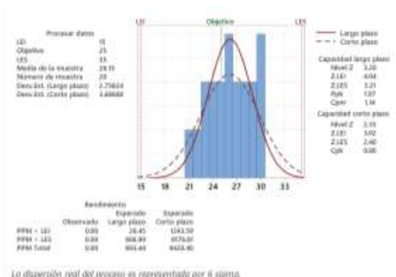
Fig. 16 Gráfica Six Sigma - CR-4 Nota. Muestra el informe de capacidad del proceso de inventario de materia prima.
