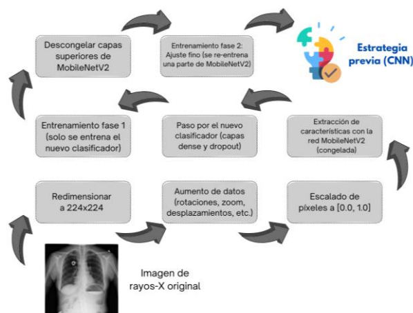
Fig. 2 Estrategia previa a la aplicación de la CNN.
