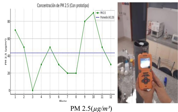
Fig. 8 Concentración de PM 2.5 con prototipo
