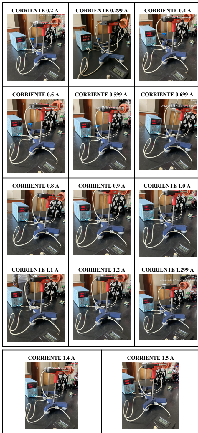
Fig 1. Mediciones para la calibración del Teslámetro con bobina estandarizada (N: 600; R: 4.2 cm)
