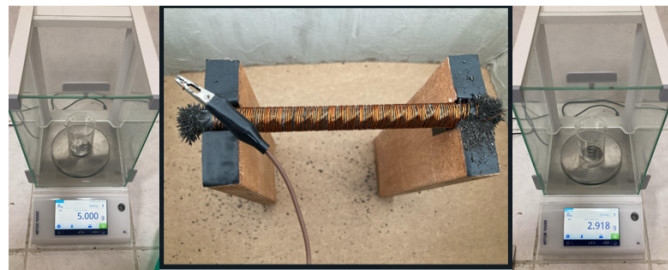
Fig 3. Proceso de la parte experimental de atracción de material particulado polimetálico mediante el prototipo de electroimán de 110 vueltas.
