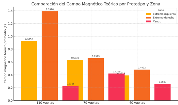
Fig 2. Comparación del campo magnético teórico promedio por prototipo y zona del núcleo
