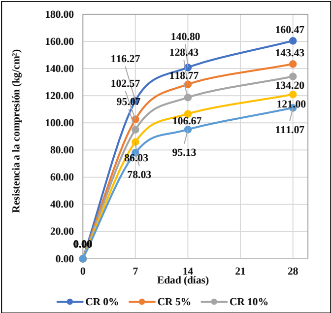
Fig. 3 Curva de resistencia a la compresión de las muestras según la adición de carcho reciclado (CR)
