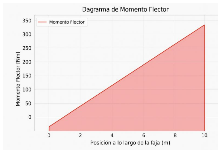
Figura 11: Momento flector
