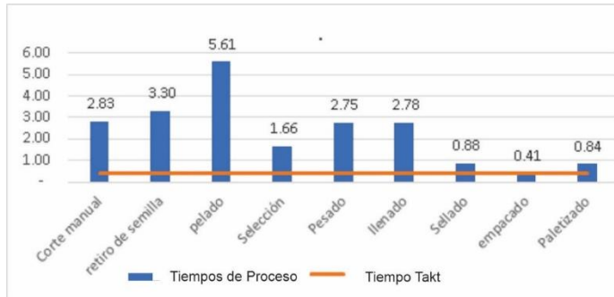
Fig. 4. Tiempos de ciclo de proceso (min) y takt time (min)
