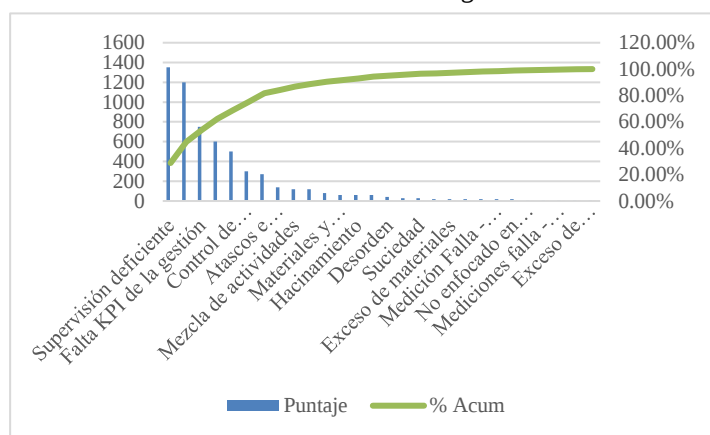
Fig. 3. Gráfico de Pareto para priorización de limitantes
