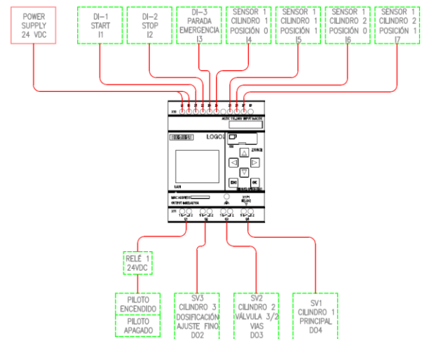
Fig. 4. Diagrama de bloques.
