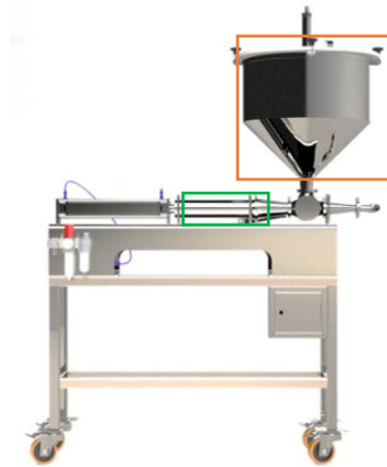
Fig. 1. Máquina dosificadora de líquidos viscosos.
