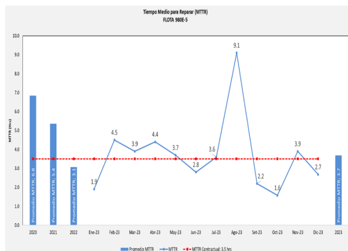
Fig. 3 Indicadores de MTTR (2023). Nota Área de mantenimiento camiones Komatsu
