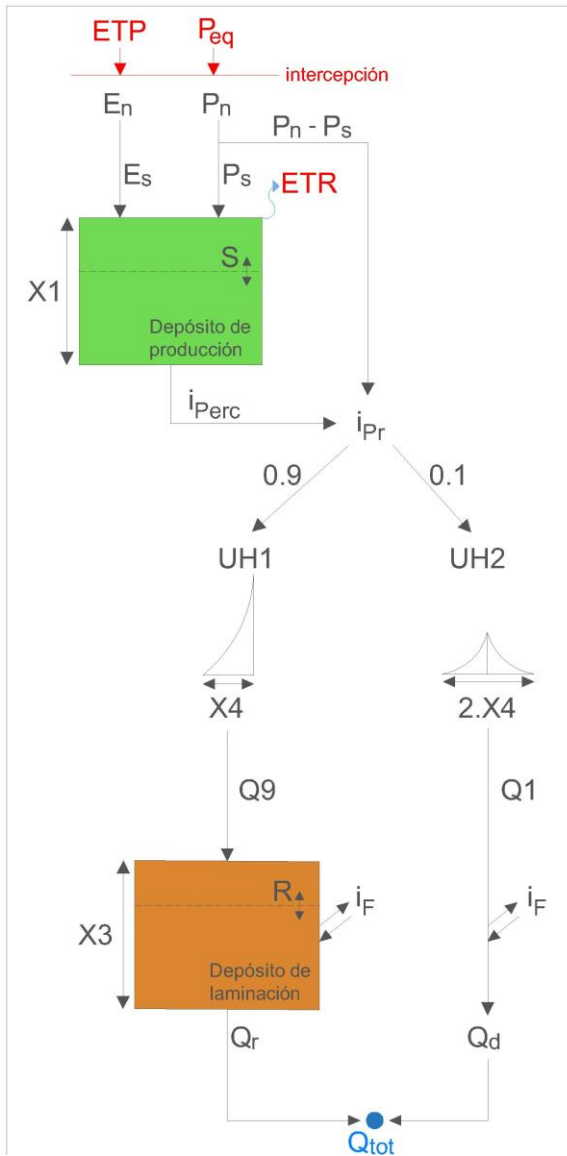
Fig. 2 GR4j modelo hidrológico (Perrin et al., 2010).
