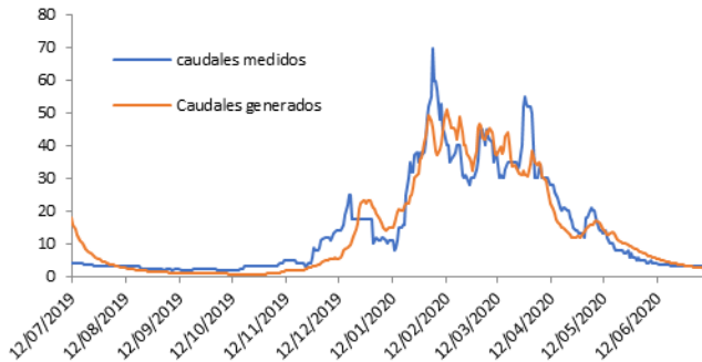
Fig. 5 Comparativa de caudales medidos (ANA) y los generados con el modelo GR4j usando datos grillados ERA5 para el periodo 1/7/2019 al 09/07/2020.
