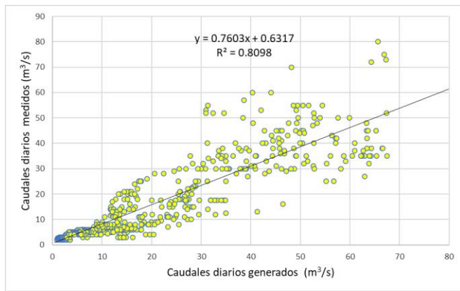
Fig. 8 Correlación R^2 entre caudales diarios generados con el método GR4j y caudales diarios medidos en el periodo 2018 - 2020.
