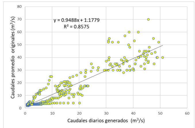
Fig. 6 Correlación R^2 entre caudales diarios generados con el método GR4j y caudales diarios medidos en el periodo de validación.
