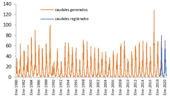
Fig. 7 Caudales a nivel diario generados con el método GR4j, en el periodo 1980 - 2020.
