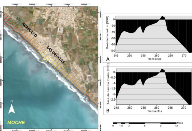
Fig. 6 Movimiento neto y tasa anual de cambio de la línea de costa de Moche de la ciudad de Trujillo en el periodo de 1985 al 2021.
