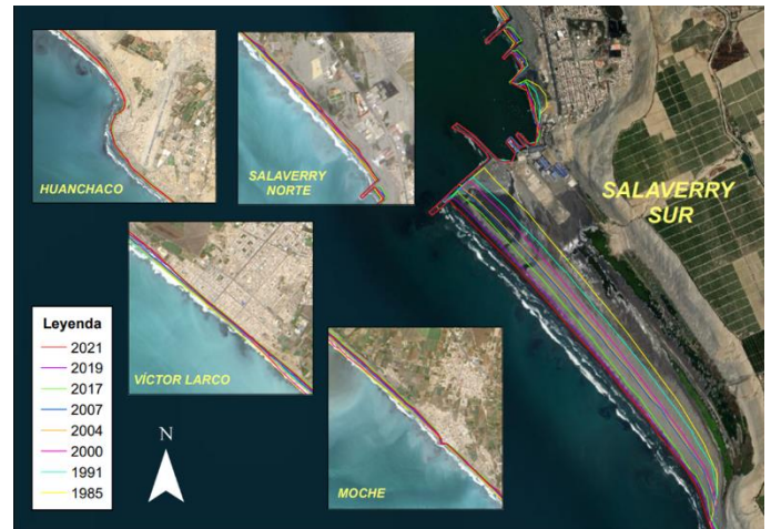
Fig. 8 Cambios de la línea de costa a causa del molón retenedor en el litoral de la ciudad de Trujillo.
