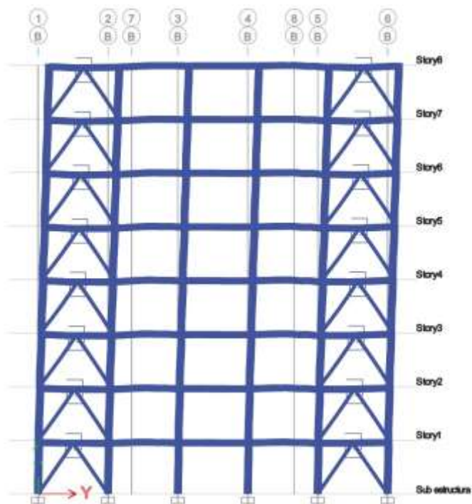
Fig. 2. Modelo estructural de ocho pisos con disipadores SLB.
