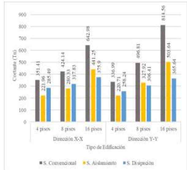
Fig. 17. Cortantes sísmicos en dirección X-X y Y-Y de las estructuras con sistema convencional, aisladores y disipadores.
