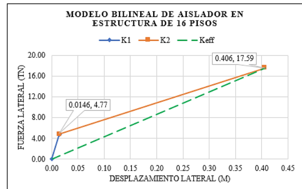
Fig. 13. Modelo bilineal de aisladores en estructura de dieciséis pisos
