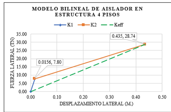
Fig. 11. Modelo bilineal de aisladores en estructura de cuatro pisos
