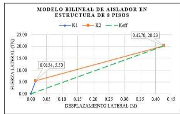
Fig. 12. Modelo bilineal de aisladores en estructura de ocho pisos
