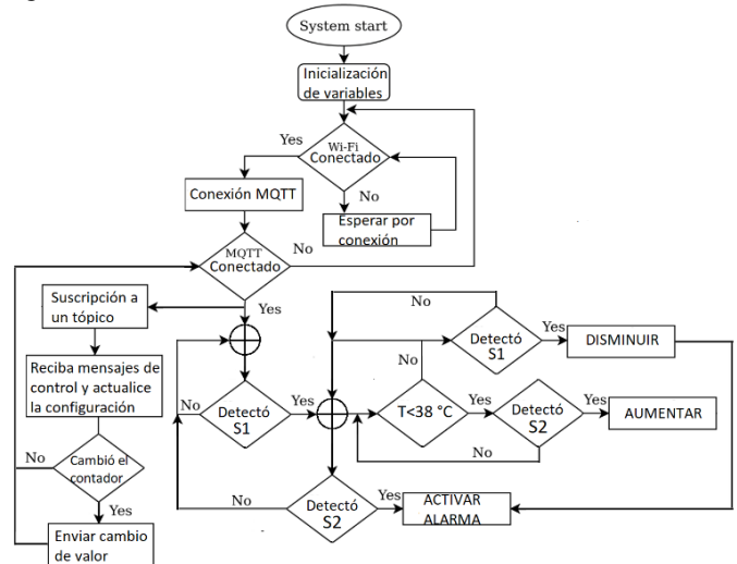
Fig. 4. Diagrama de Flujo
