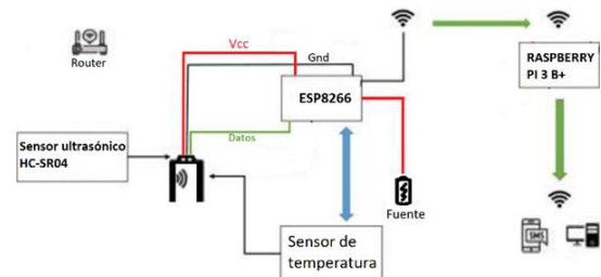
Fig. 1 Estructura general del sistema de conteo y medición de temperatura de las personas
