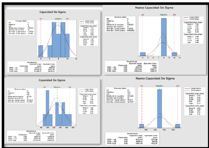
Figura 46 SIX-SIGMA de la CR5-A-B antes y después
