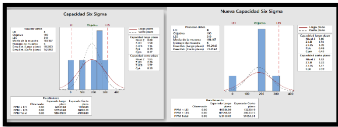
Figura 44 SIX-SIGMA de la CR3 antes y después
