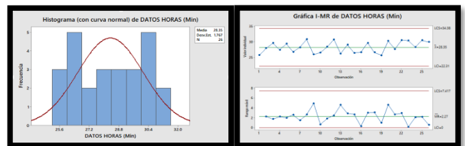
Figura 9 Histograma y Gráfica de Control (C) de CR1
