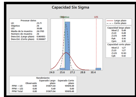
Figura 17 Capacidad Six-Sigma de CR1
