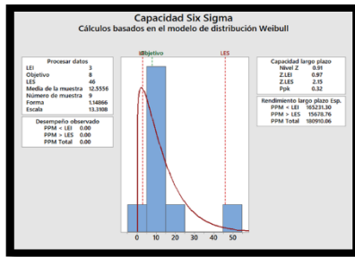
Figura 19 Capacidad Six-Sigma de CR2
