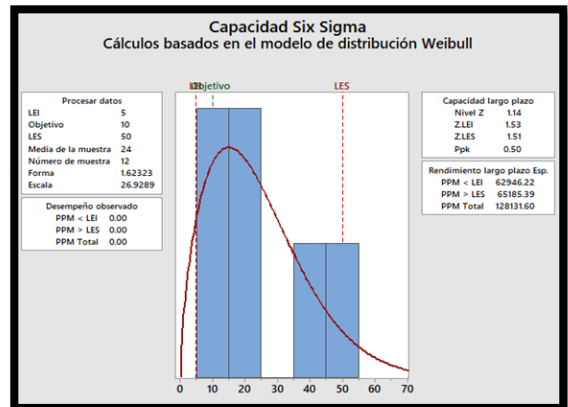
Figura 22 Capacidad Six-Sigma de CR4
