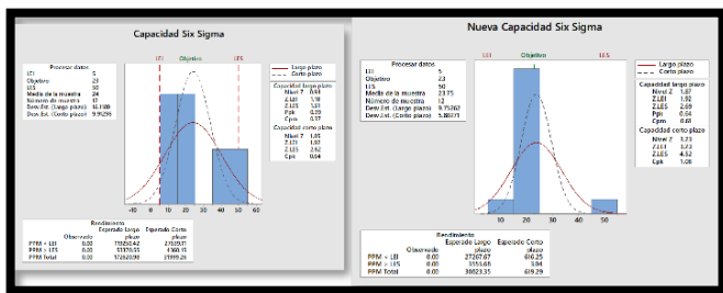
Figura 45 SIX-SIGMA de la CR4 antes y después
