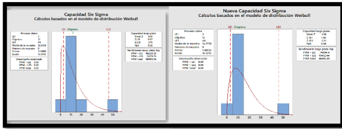
Figura 43 SIX-SIGMA de la CR2 antes y después
