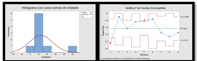
Figura 10 Histograma y Gráfica de Control (P) de CR2
