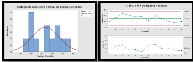
Figura 13 Histograma y Grafica de Control (C) de CR5B
