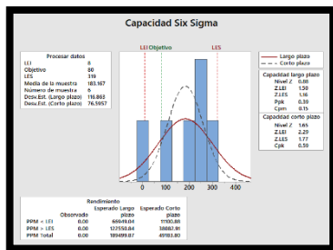
Figura 21 Capacidad Six-Sigma de CR3
