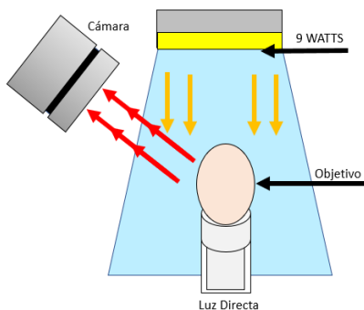
Figura 1. Sistema controlado de iluminación para examinación de las muestras de huevos
