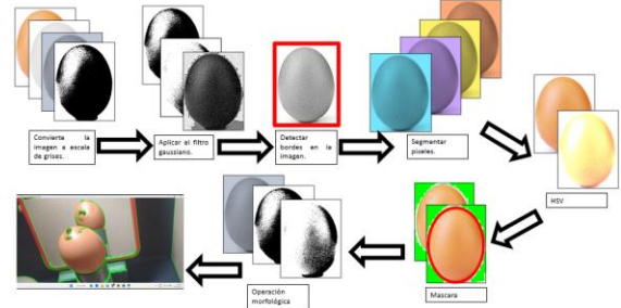
Figura 2: Funcionamiento del algoritmo
