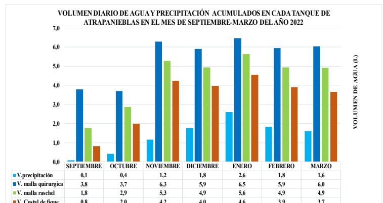
Fig. 3: Se muestra el volumen acumulado del agua captado en los tanques y las precipitaciones en cada malla: Tela quirúrgica, Raschel y costal de fique.
