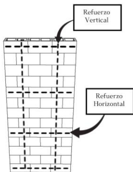
Fig. 4 Refuerzo horizontal y vertical basado en [7]
