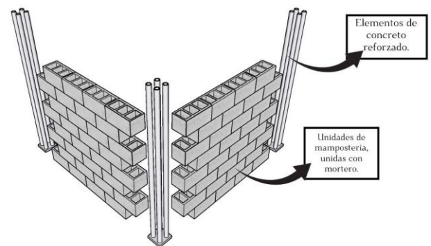
Fig. 1 Mampostería simple basado en [3]
