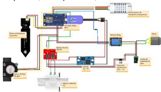
Fig. 2 Esquema de conexión de sensores y actuadores. Fuente: Elaboración propia.
