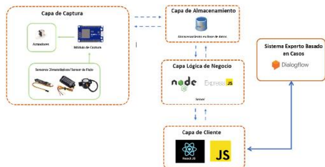
Fig. 1 Arquitectura del sistema. Fuente: Elaboración Propia.
