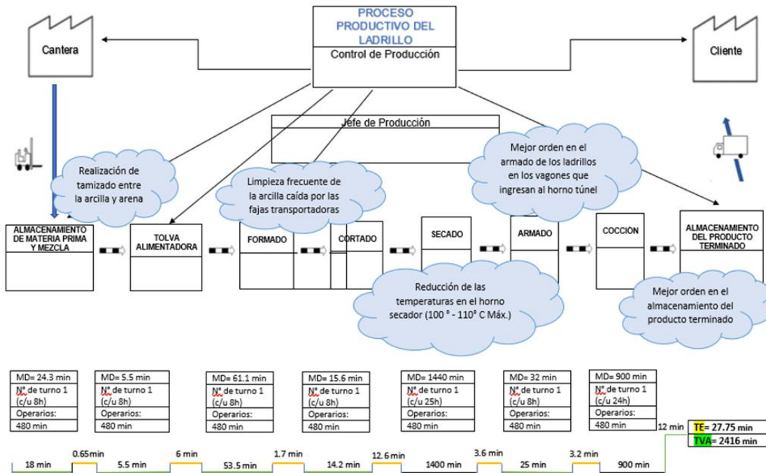
FIGURA III VSM POST APLICACIÓN DE LEAN MANUFACTURING DEL PROCESO PRODUCTIVO DE LA EMPRESA
