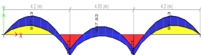
Fig. 4 Diagrama de momentos – Envolvente
