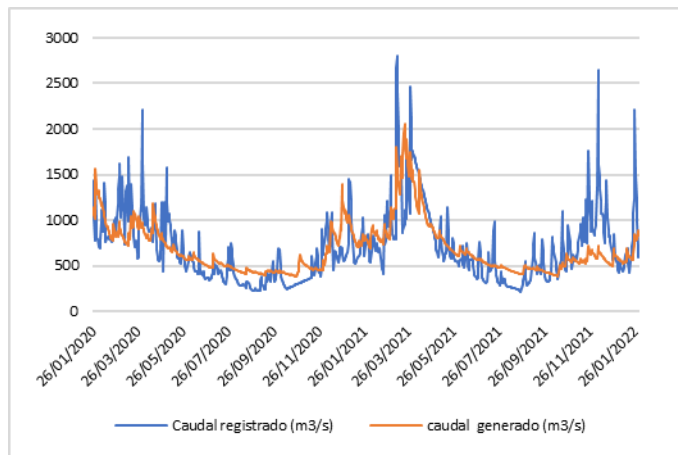
Fig. 7 Comparativa de caudales diarios medidos (ANA) y caudales generados (GR4j) para la cuenca Huayabamba en el proceso de validación entre el 31/12/19 al 22/2/2022
