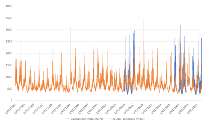
Fig. 9 Comparativa diaria de caudales medidos (ANA) y caudales generados (GR4j) para la cuenca Huayabamba en el periodo entre 02/01/1981 hasta el 09/07/2020
