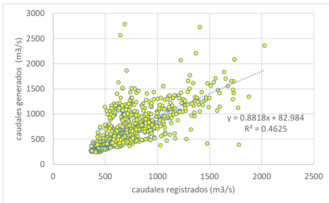
Fig. 6 Correlación del R^2 entre caudales diarios medidos (ANA) y caudales generados (ERA 5) para el periodo de calibración
