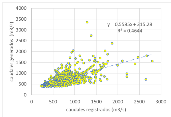
Fig. 8 Correlación del R^2 Comparativa de caudales diarios medidos (ANA) y caudales generados (ERA5) para la cuenca Huayabamba en el proceso de validación entre el 31/12/19 al 22/2/2022
