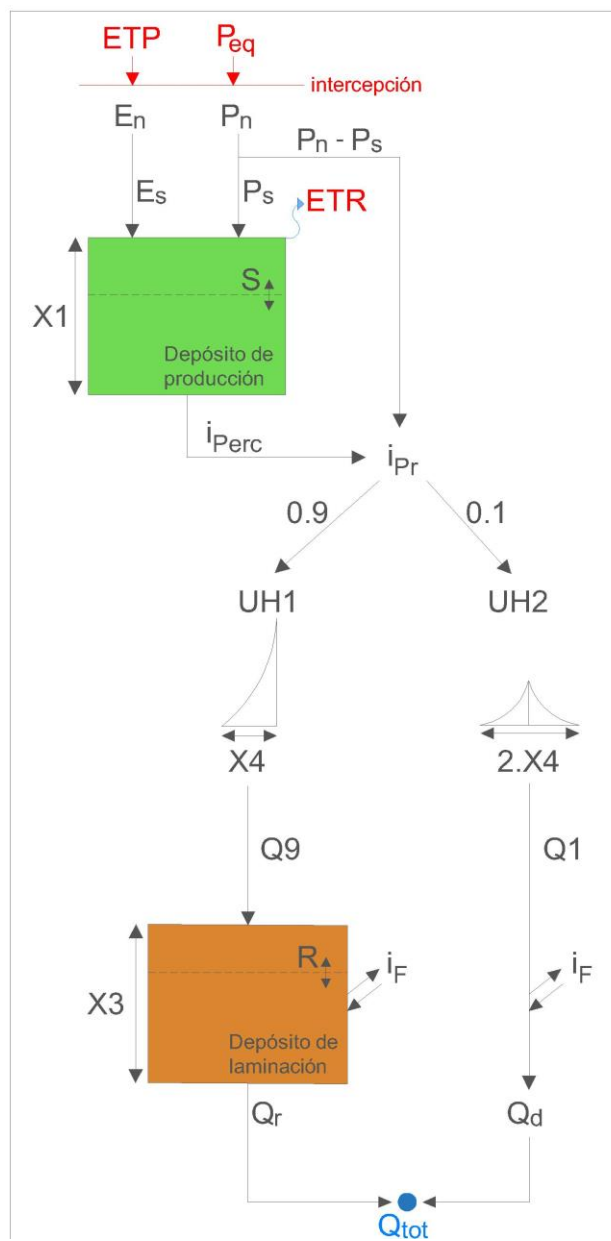
Fig. 4 Modelo de precipitación – escorrentía GR4j (Perrin et al., 2010).
