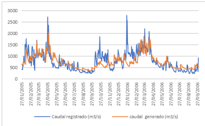
Fig. 5 Comparativa de caudales diarios medidos (ANA) y caudales generados (GR4j) para la cuenca Huayabamba en el proceso de calibración entre el 01/10/2001 hasta el 30/09/2004
