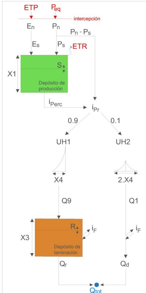
Fig. 5 GR4j modelo hidrológico (Perrin et al., 2010) [8].
