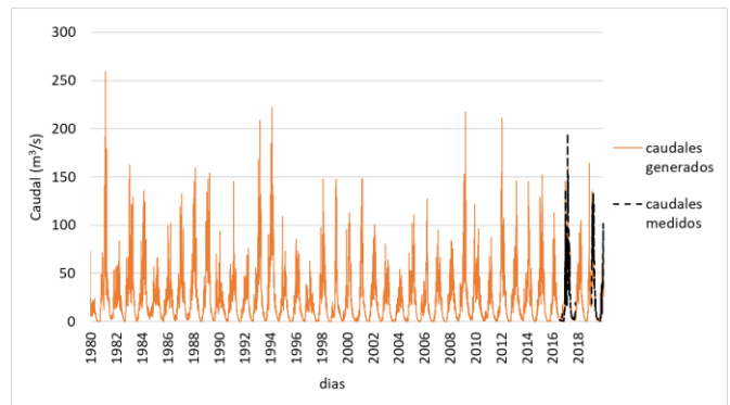
Fig. 8 Comparativa diaria de caudales medidos (ANA) y caudales promedio diarios con GR4j generados para la cuenca del río Crisnejas hasta la estación hidrométrica Puente Crisnejas entre los días 02/01/1979 hasta el 09/07/2020
