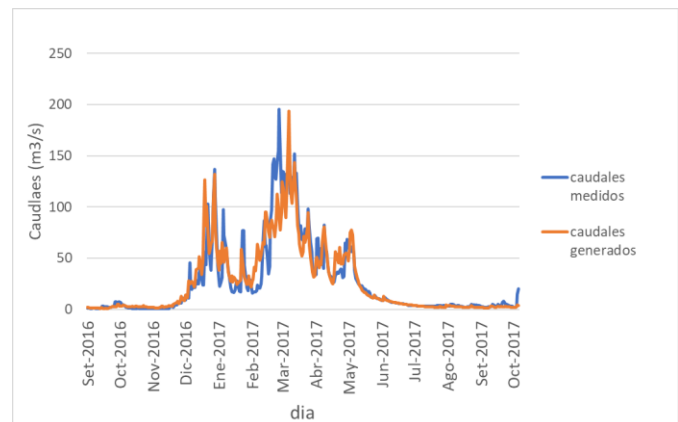
Fig. 3 Comparativa entre los caudales promedio originales (ANA) y caudales promedio diarios con GR4j generados en el proceso de calibración
