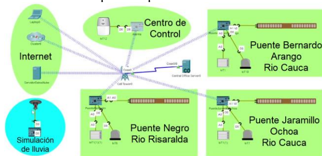
Figura 3. Simulación de las estaciones en Cisco Packet Tracer
