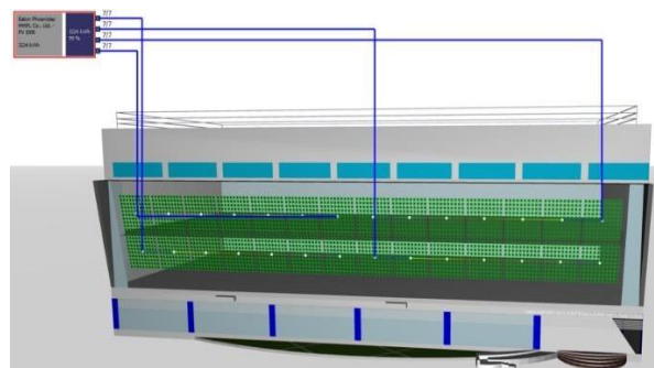
Fig. 6 Conexión de paneles X5 e inversor Eathon Phoenixtec con conexión a la red
