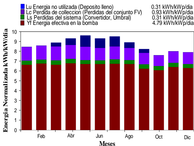
Fig. 5 Simulación del sistema eléctrico fotovoltaico usando la bomba seleccionada
