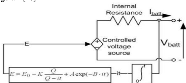
Fig. 4 Modelo de Shepherd
