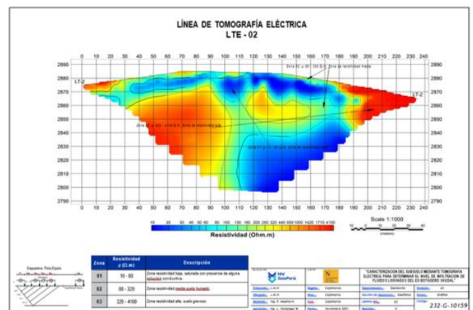
Figura 5. Perfil de resistividades LTE - 02
