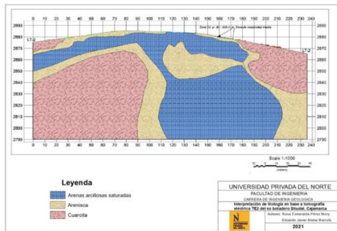
Figura 7. Interpretación litológica LTE - 02
