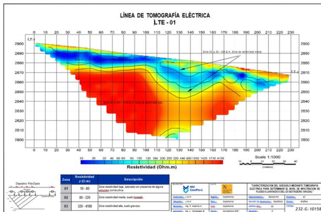
Figura 4. Perfil de resistividades LTE - 01
