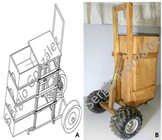
Fig. 3. Vista isométrica del concepto a desarrollar. B. Modelado finalizado.
