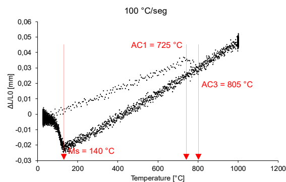
Fig. 3 Curvas de dilatación vs temperatura, para diferentes velocidades de calentamiento
