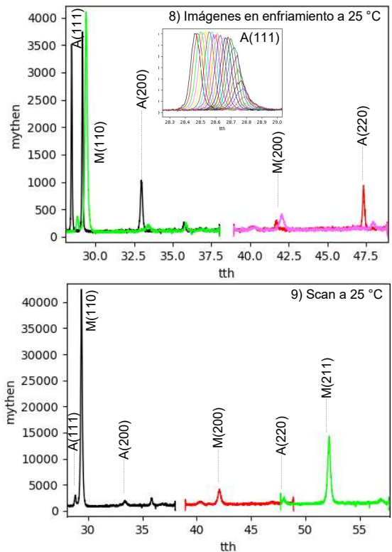
Fig. 6 a: Etapa 7, b: Etapa 8, c: Etapa 9 en el ciclo S+R. En b y c: negro y rojo: inicio, verde y rosa: fin
