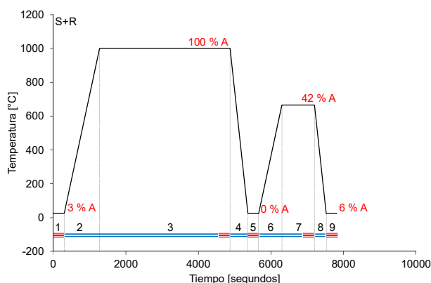
Fig. 7 Contenido de austenita medido en las diferentes etapas para el tratamiento S+R
