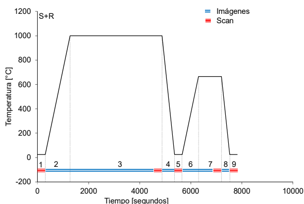
Fig. 2 Tratamientos térmicos: S+R: solubilizado + revenido intercrítico
