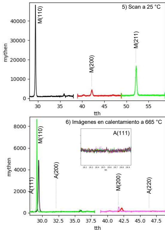
Fig. 5 a: Etapas 4, b: Etapa 5, c: Etapa 6 en el ciclo S+R. En b y c: negro y rojo: inicio, verde y rosa: fin
