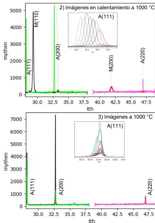
Fig. 4 a: Etapa 1, b: Etapa 2, c: Etapa 3 en el ciclo S+R. En b y c: negro y rojo: inicio, verde y rosa: fin
