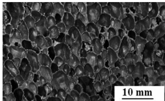
Fig. 6 – Espuma de Aluminio de poro cerrado [25]
