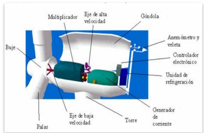
Fig. 4 – Góndola del generador eólico [20]
