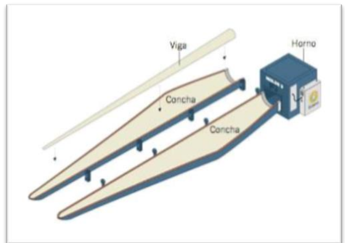
Fig. 5 – Estructura central y cubiertas externas de una pala eólica [33]
