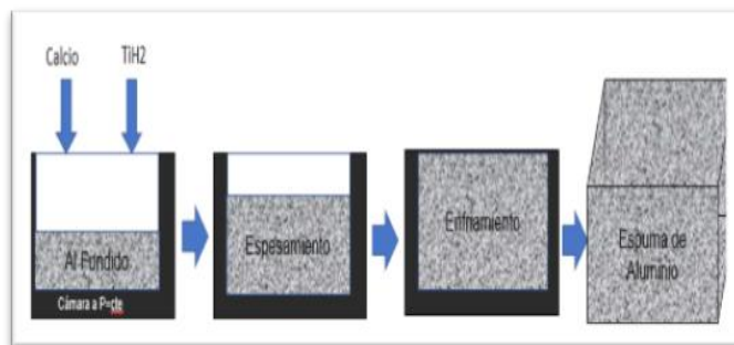
Fig. 9 – Fabricación de espumas de aluminio por método Alporas
