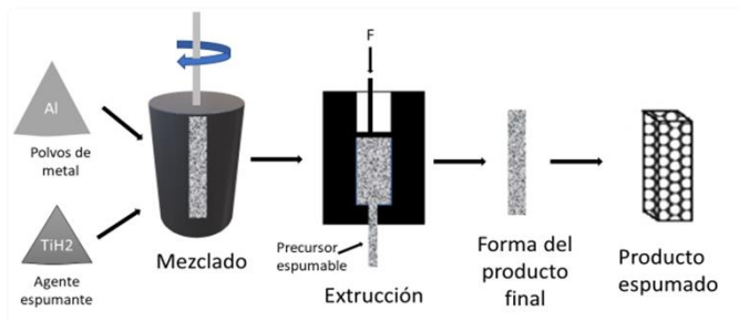
Fig. 11 – Fabricación de espumas de aluminio por métodos de Pulvimetalurgia
