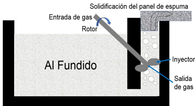
Fig. 8 – Fabricación de espumas de aluminio por método Alcan
