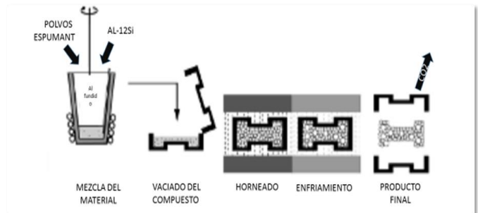
Fig. 12 – Fabricación de espumas de aluminio por método Foamcarp
