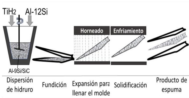
Fig. 10 – Fabricación de espumas de aluminio por método Formgrip
