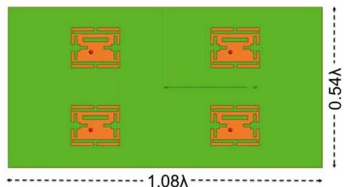
Fig. 2. La estructura base o de referencia donde se muestra las cuatro antenas operando a 2.6GHz. Longitud de onda - \lambda .
