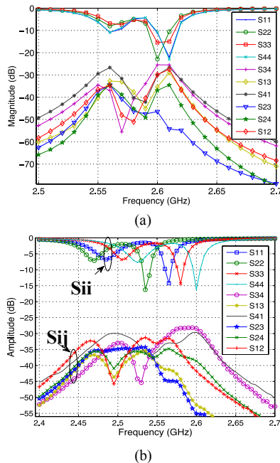
Fig. 6. Parámetros S del arreglo propuesto. (a) Simulados, y (b) Medidos.
