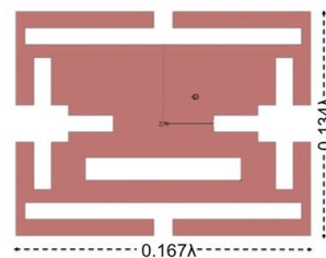
Fig. 1. Diseño de la antena tipo patch miniaturizada utilizando slots para operar a 2.6 GHz.
