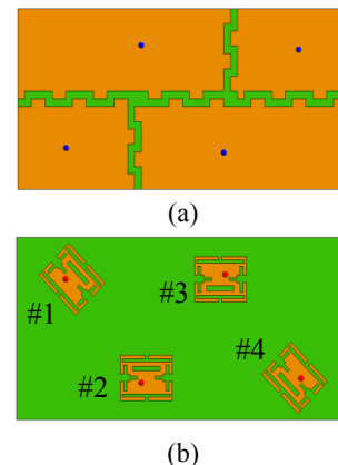
Fig. 5. Diseño final del arreglo MIMO. (a) 4-antenna sobre el sustrato dieléctrico (PCB). (b) GND modificado con slots corrugados (pequeños triángulos).
