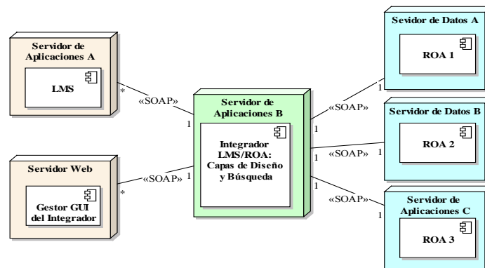
Figura 6. Despliegue de los componentes de la arquitectura del Integrador LMS/ROA
