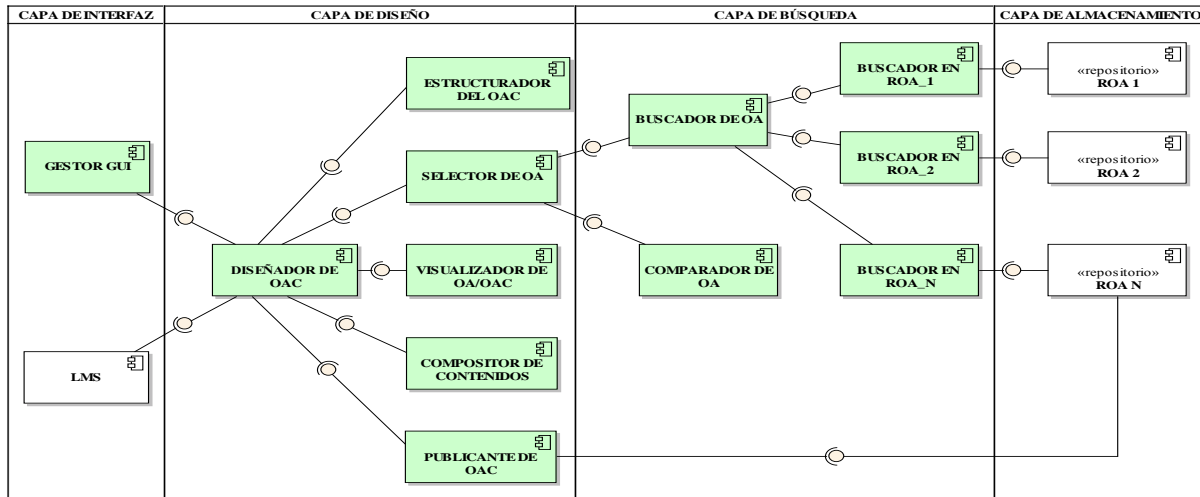
Figura 5. Servicios web que conforman la arquitectura del Integrador LMS/ROA
