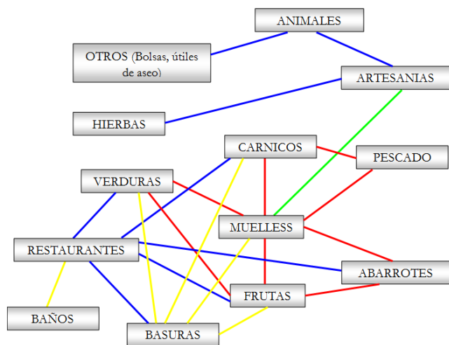
Figura 4. Diagrama de Planificación Sistemática de la Disposición de Espacio.
