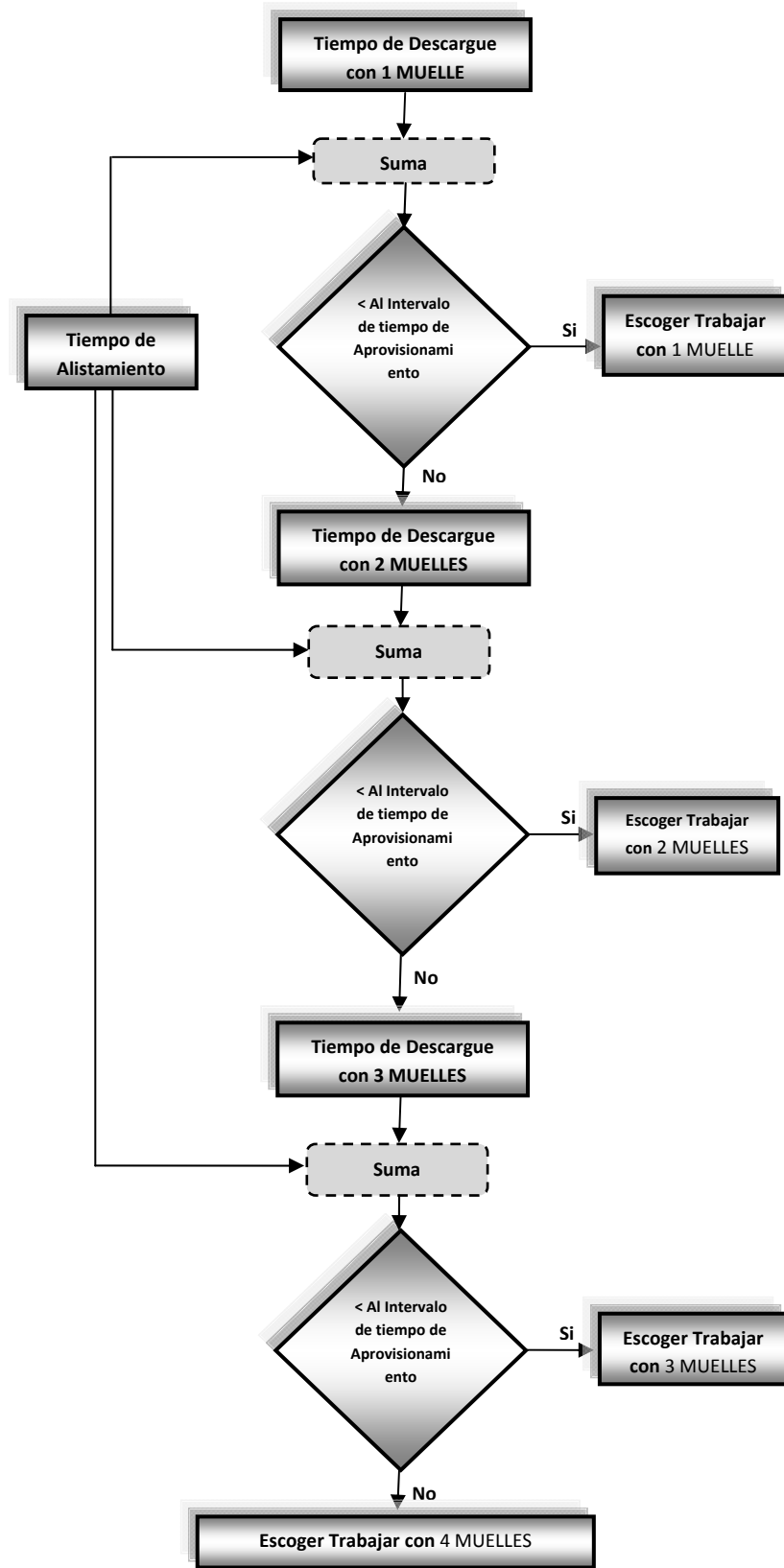
Figura 3. Algoritmo para la selección del Número de Muelles
