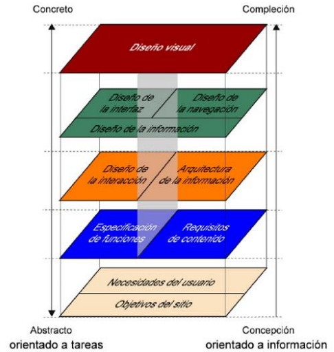
Fig. 11 - Elementos de Experiencia de usuario
