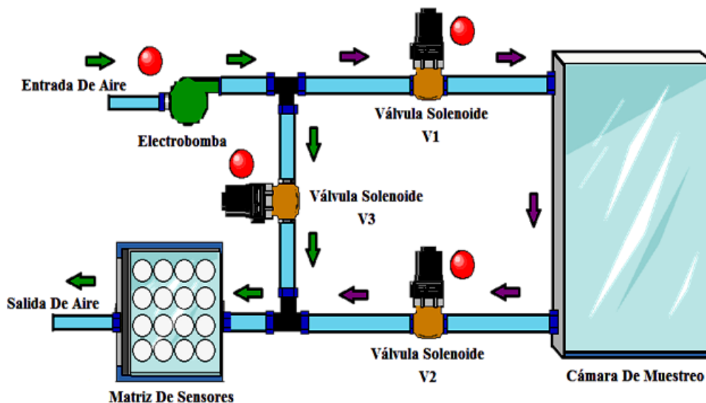
Figura 1: Diseño del equipo multisensor
