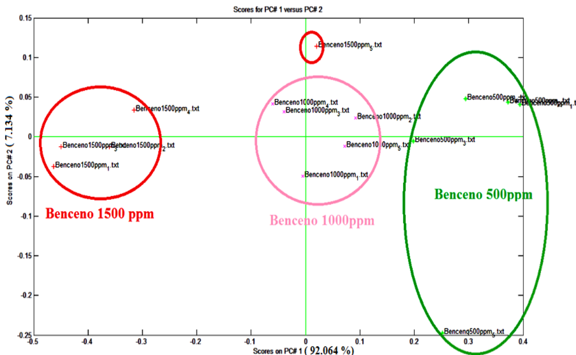
Figura 3: Resultado del análisis PCA con los grupos de medidas de Benceno a: 500 ppm, 1000 ppm y 1500 ppm.
