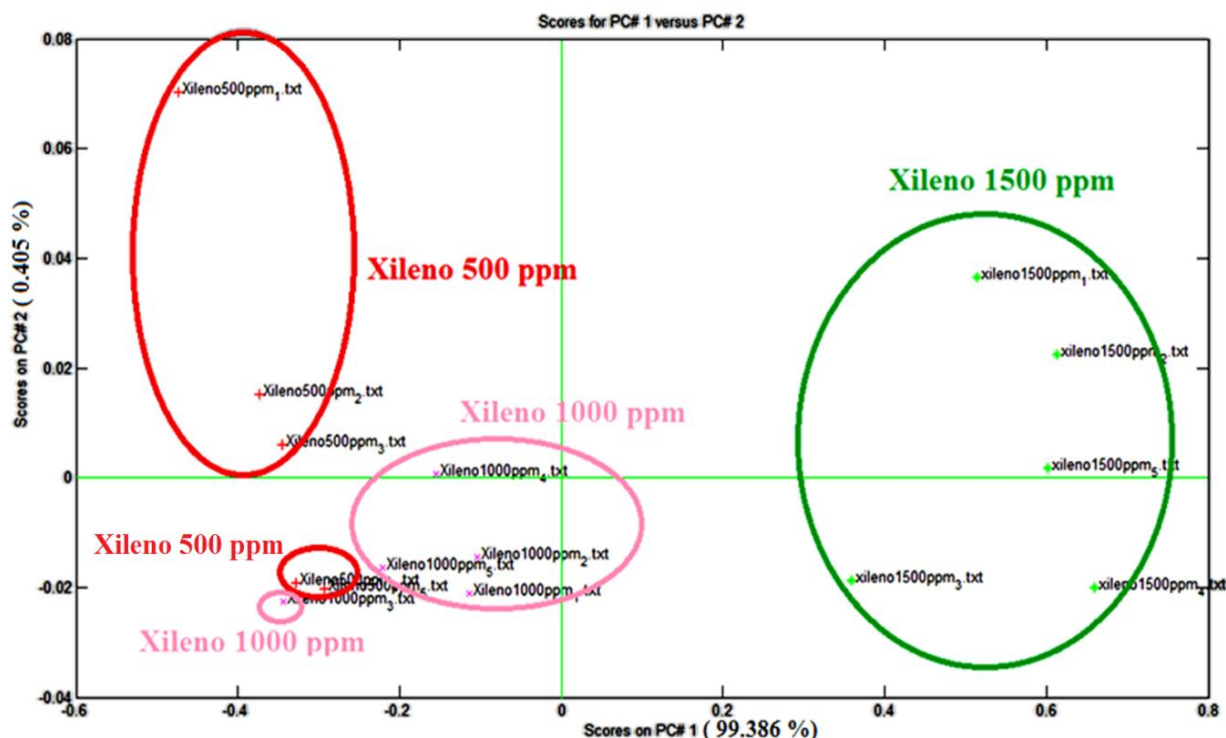
Figura 5: PCA de las medidas de Xileno a: 500 ppm, 1000 ppm y 1500 ppm.
