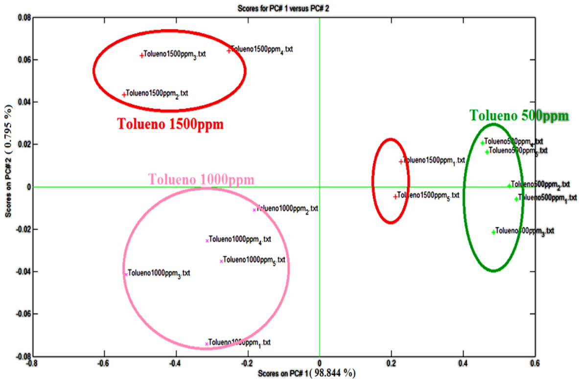
Figura 4: Gráfica PCA con las medidas de concentración de Tolueno a: 500 ppm, 1000 ppm y 1500 ppm.
