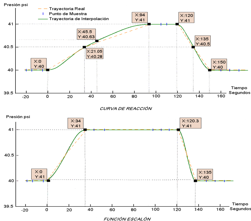
Figura N° 2. Curva de reacción del proceso o respuesta escalón de circuito abierto.
