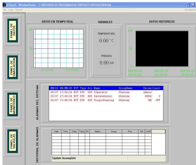
Figura N° 9. Pantalla de datos del proceso de esterilización.
